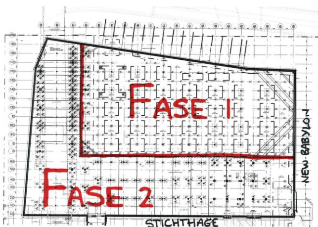
Figuur 1. Overzichtstekening ontgraving en bemaling
