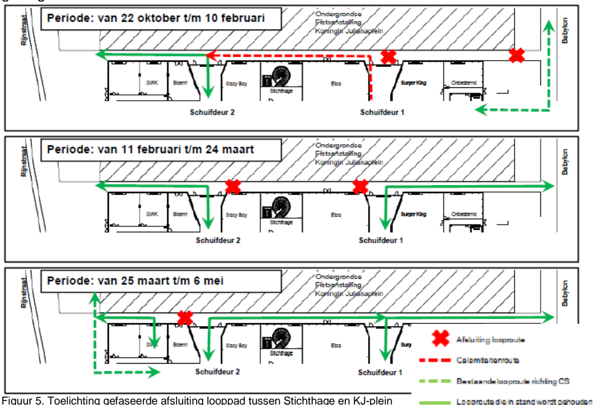
Figuur 5. Toelichting gefaseerde afsluiting looppad tussen Stichthage en KJ-plein
