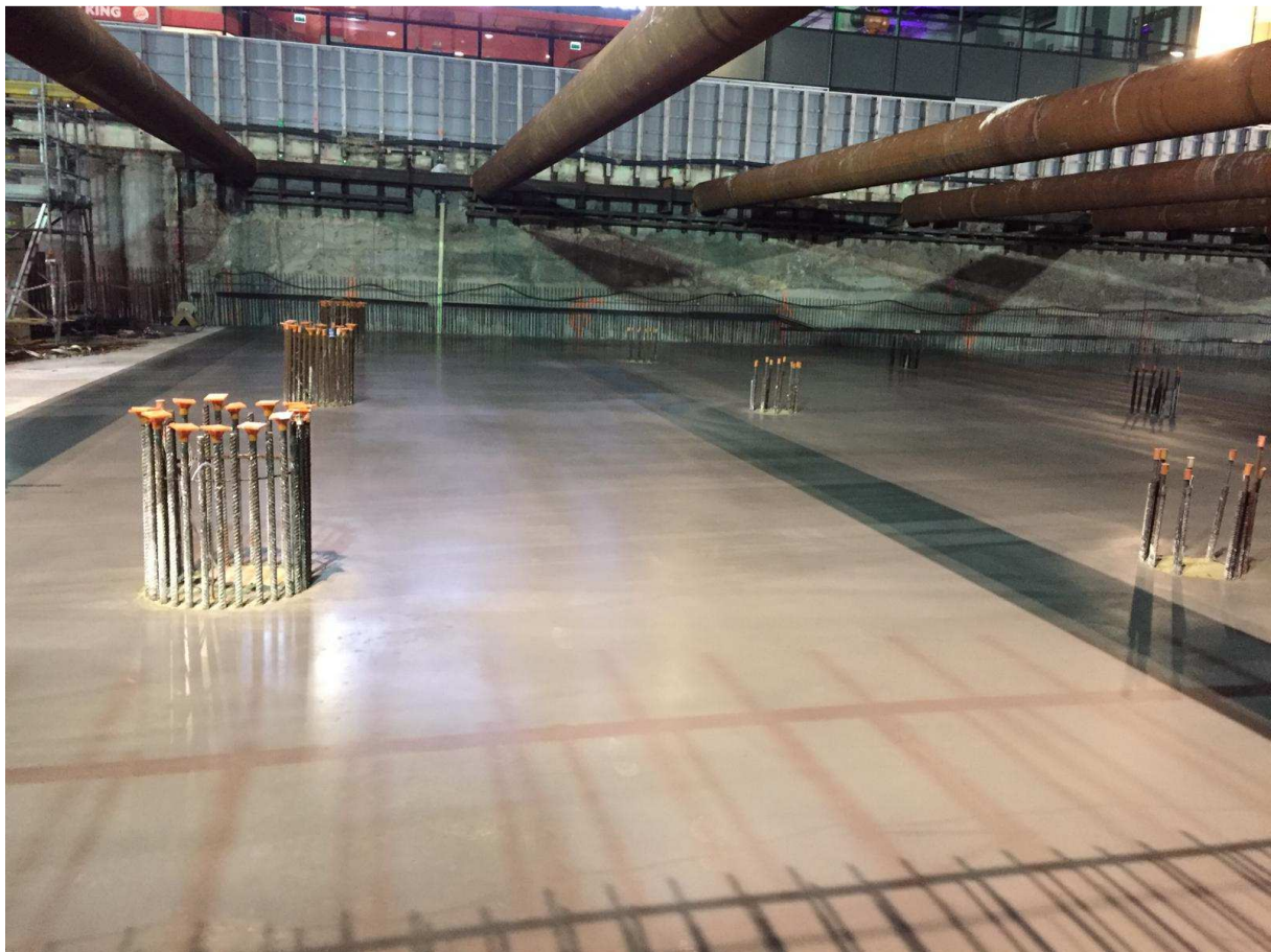
Figuur 3. Net gestorte vloer met de uitstekende stalen pennen (wpeningsstekken).
