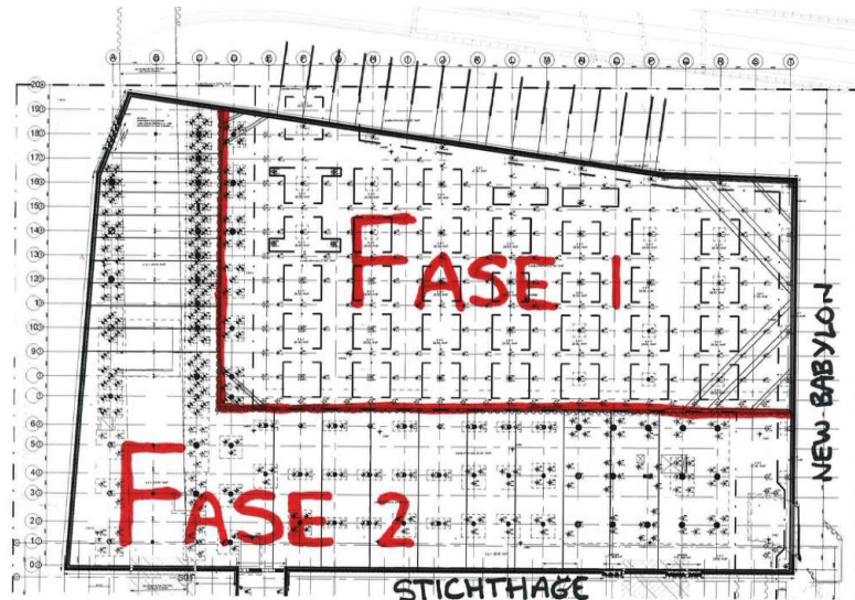
Afbeelding 2. Overzichtstekening ontgraving en bemaling
